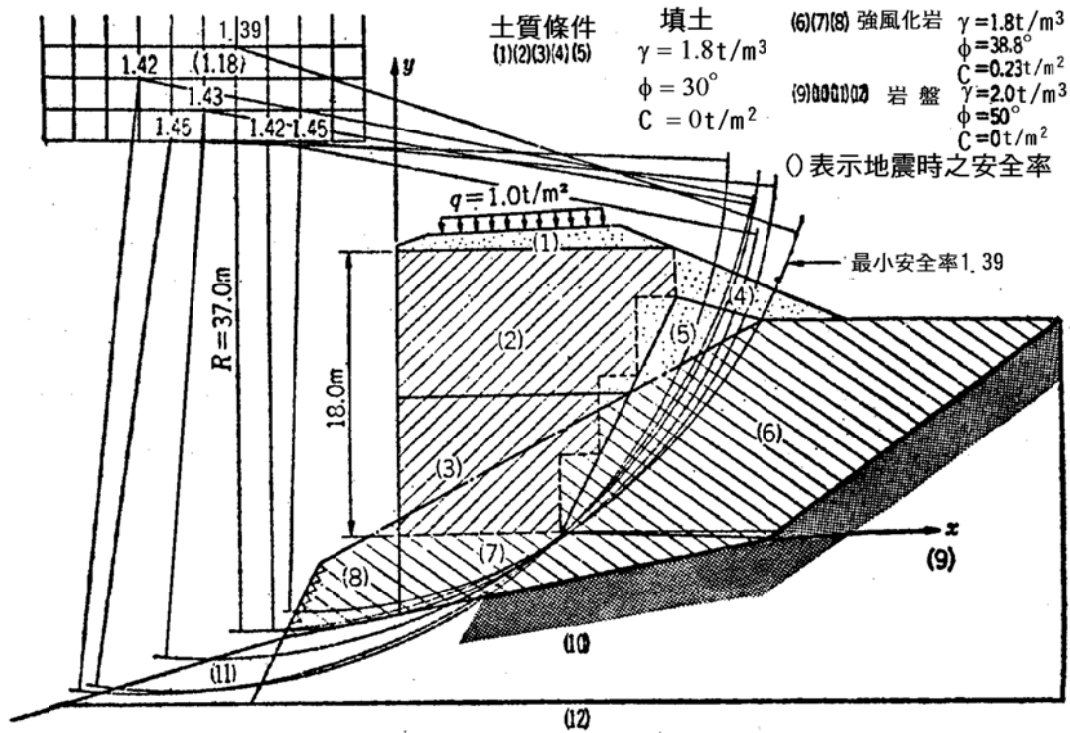
圖(m) 圓弧轉動破壞檢討實例
