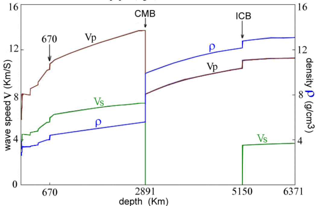
Fig. 1 The data of PREM : \rho : density ; V : velocity.
