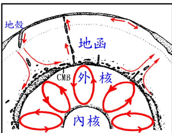
雙循環地球內部構造模式示意圖
