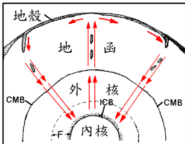
單循環地球內部構造模式示意圖
