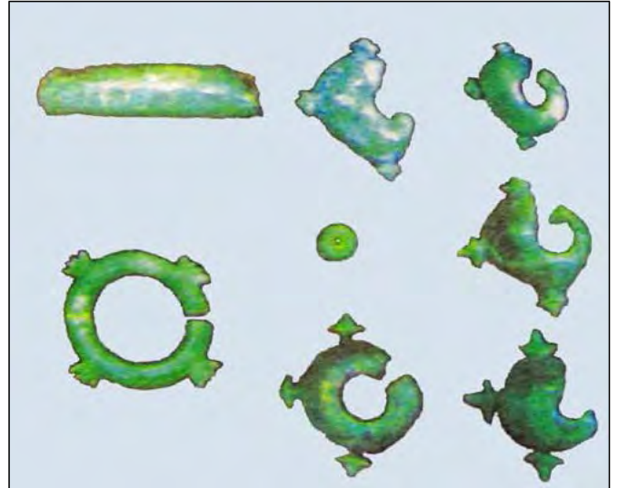
巴丹群島阿納羅的玉器被證明為「豐田玉」
